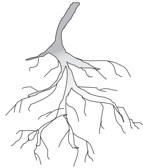
Dicot Root
